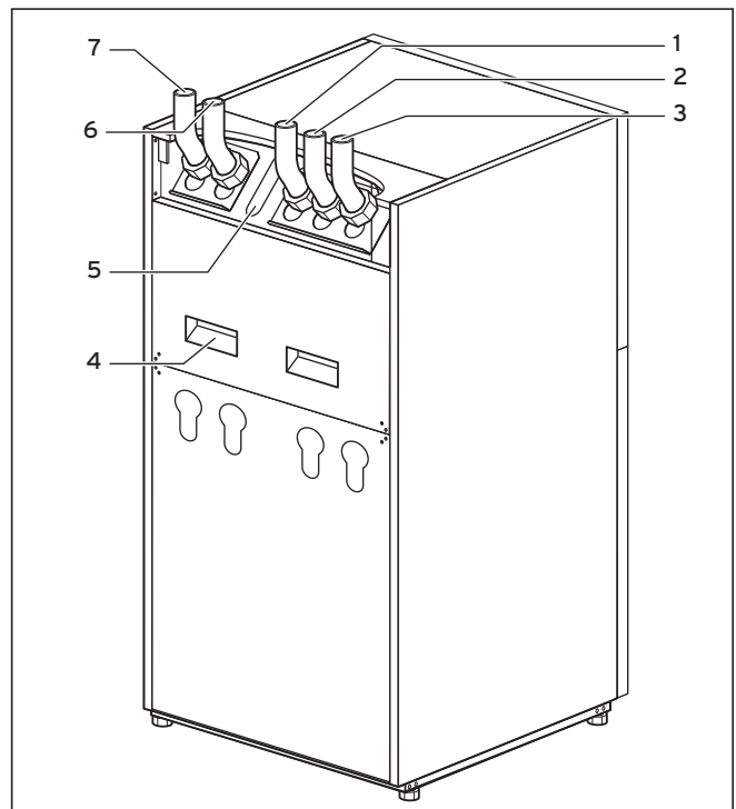
Fig. 4.4 Vue arrière
