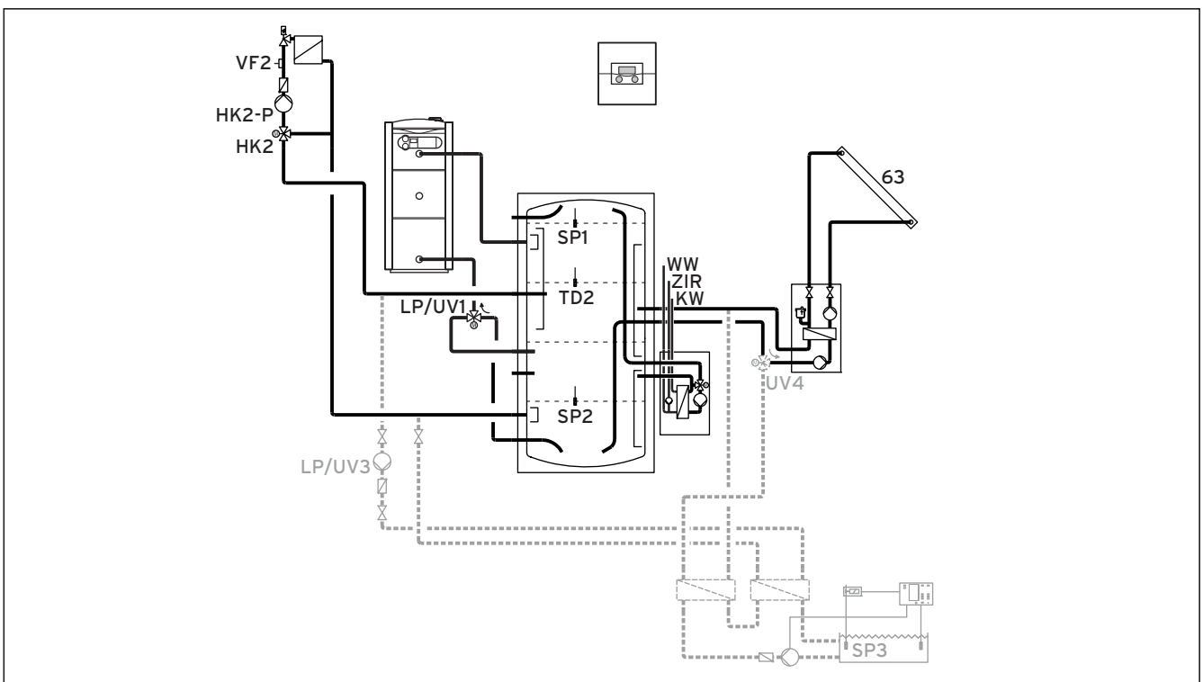
Fig. 5.37 Schéma hydraulique 9.2
