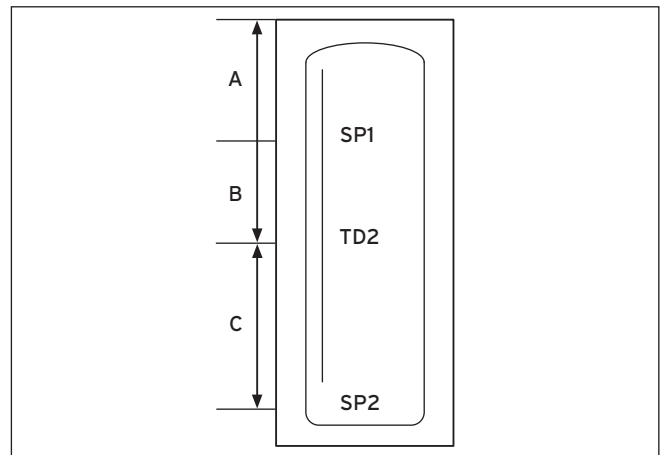
Fig. 5.48 Affectation des capteurs SP1, TD2 et SP2 dans le ballon d'accumulation
