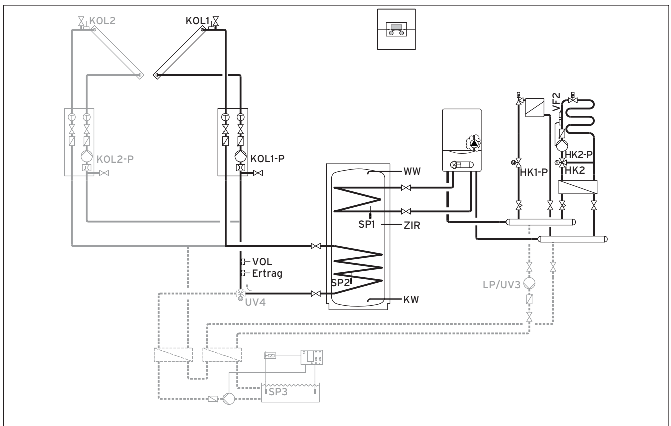
Fig. 5.13 Schéma hydraulique 3.2
