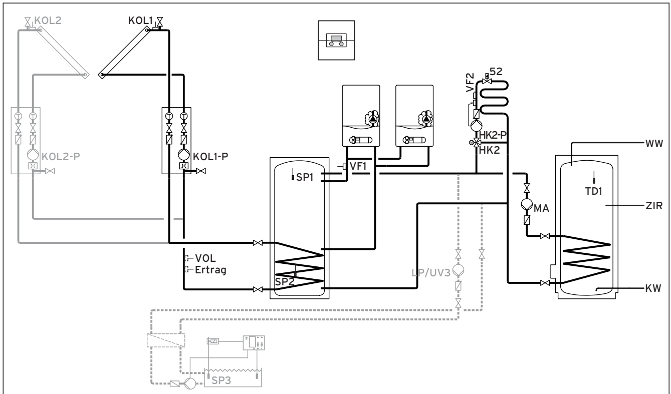
Fig. 5.25 Schéma hydraulique 5.2
