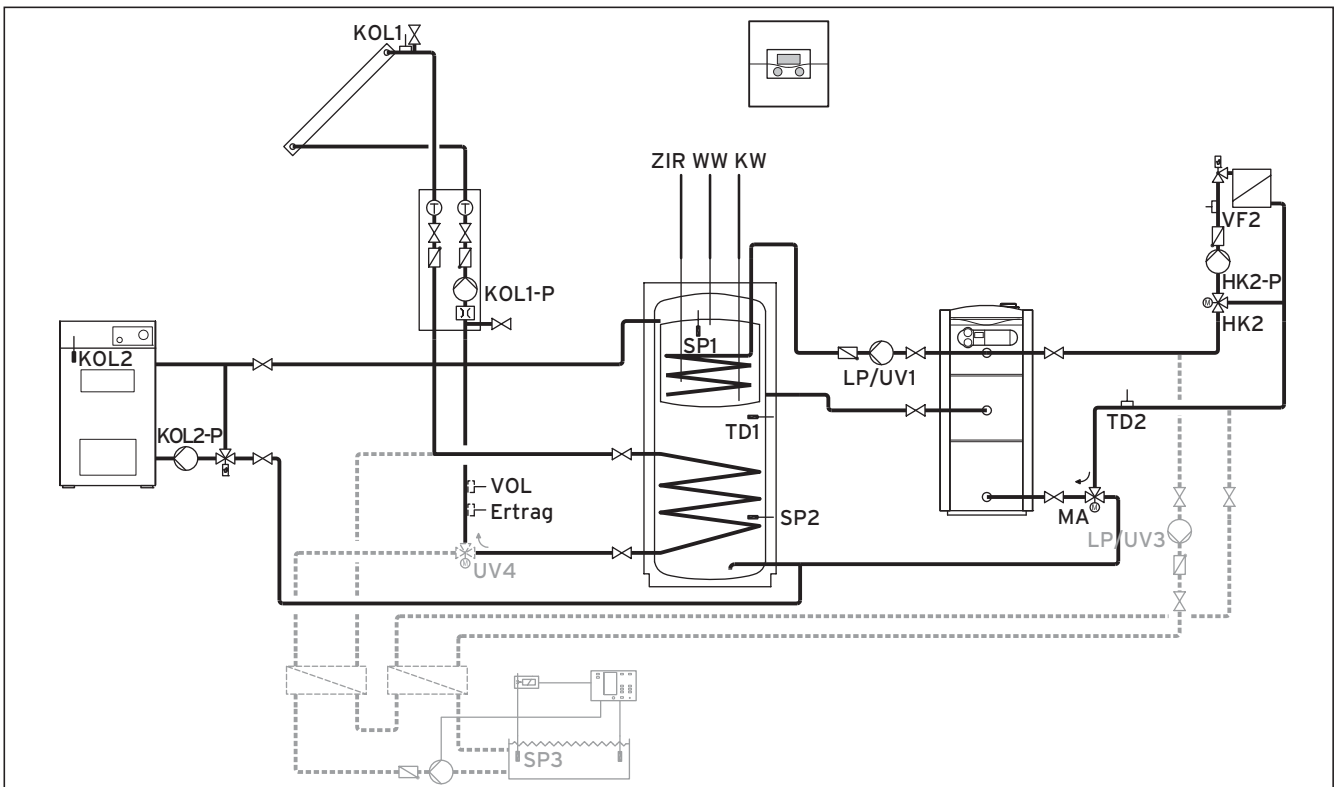
Fig. 5.19 Schéma hydraulique 4.1
