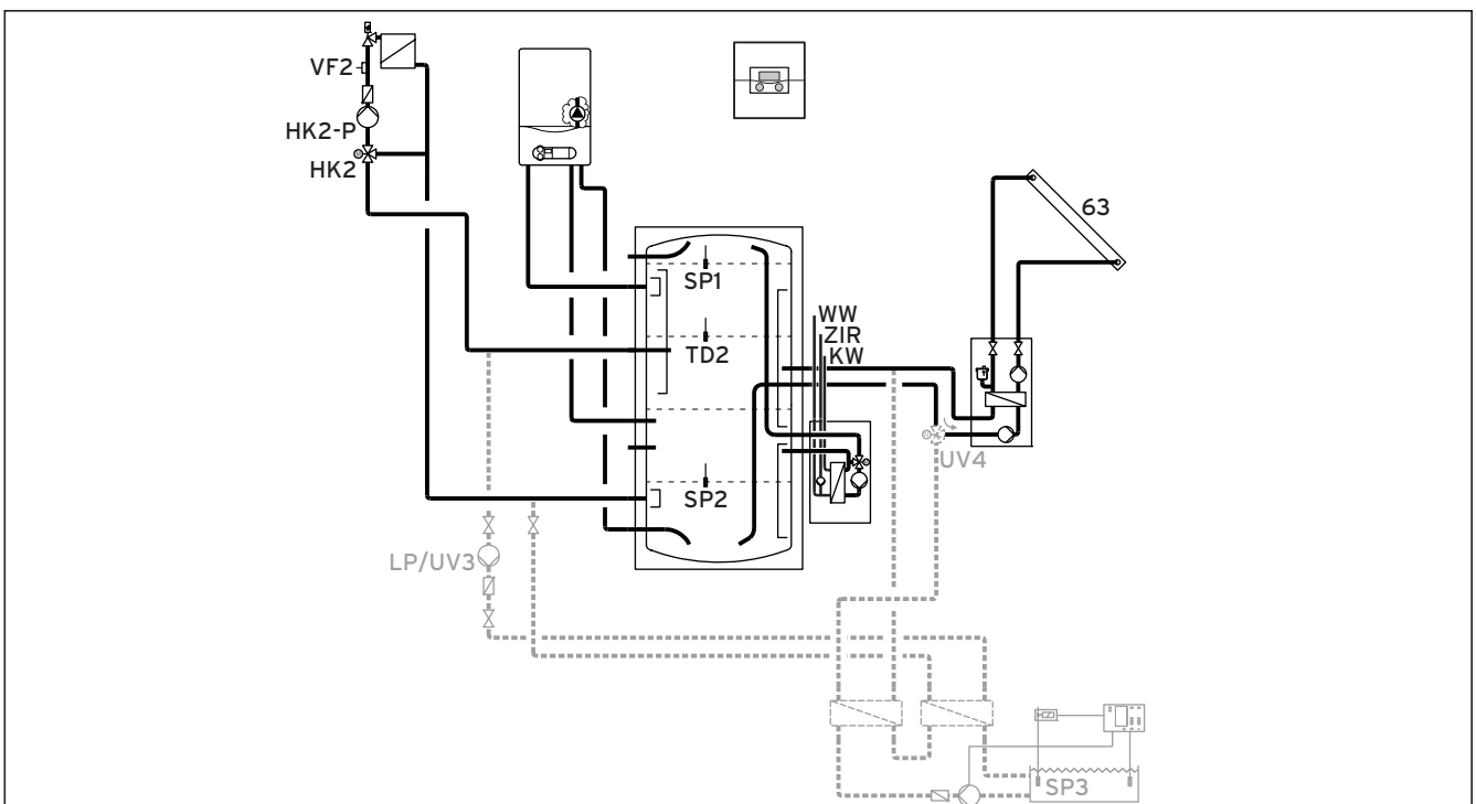
Fig. 5.35 Schéma hydraulique 9.1
