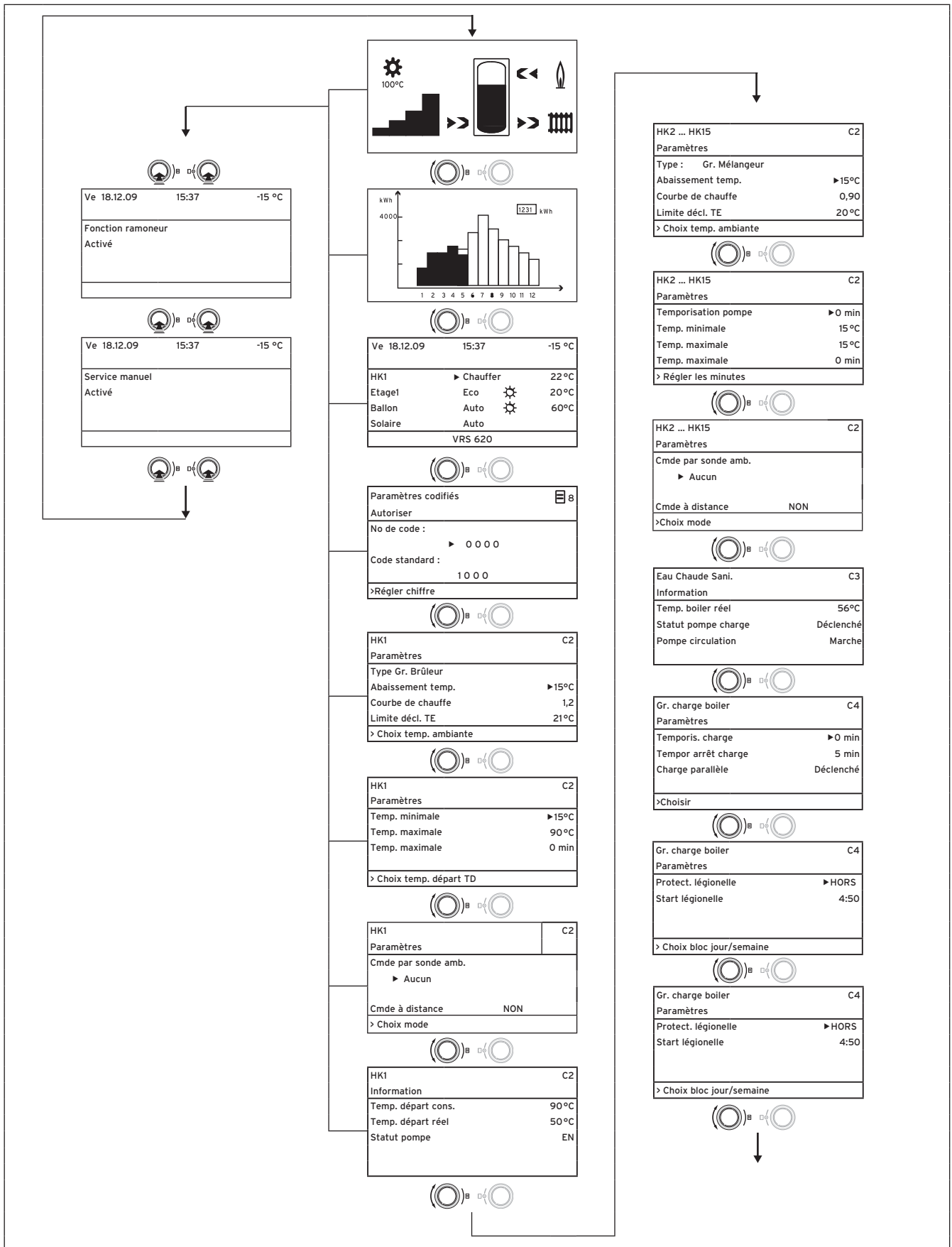
Fig. 3.7 Structure de menu du niveau réservé à l'installateur
