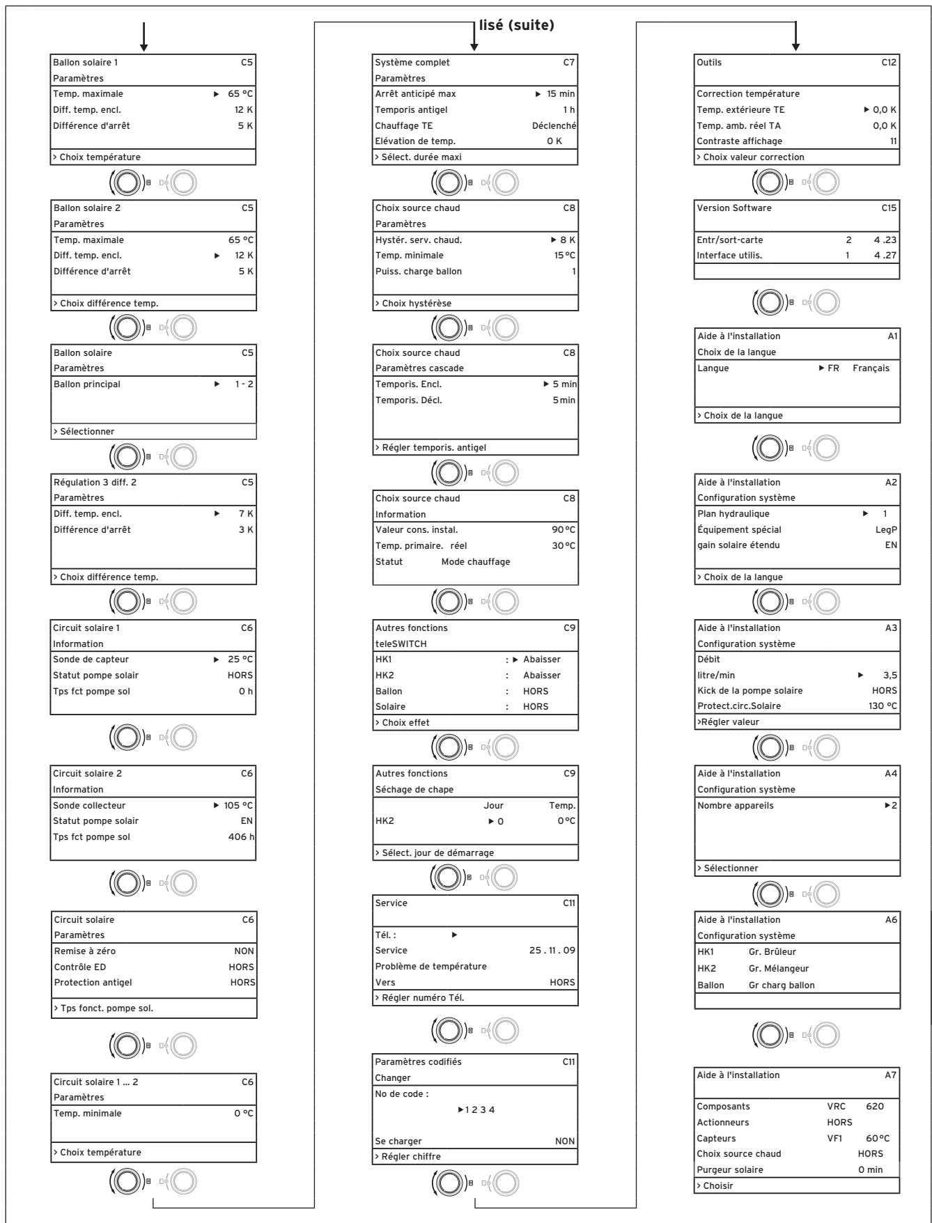
Fig. 3.7 Structure de menu du niveau de l'installateur spécia-
