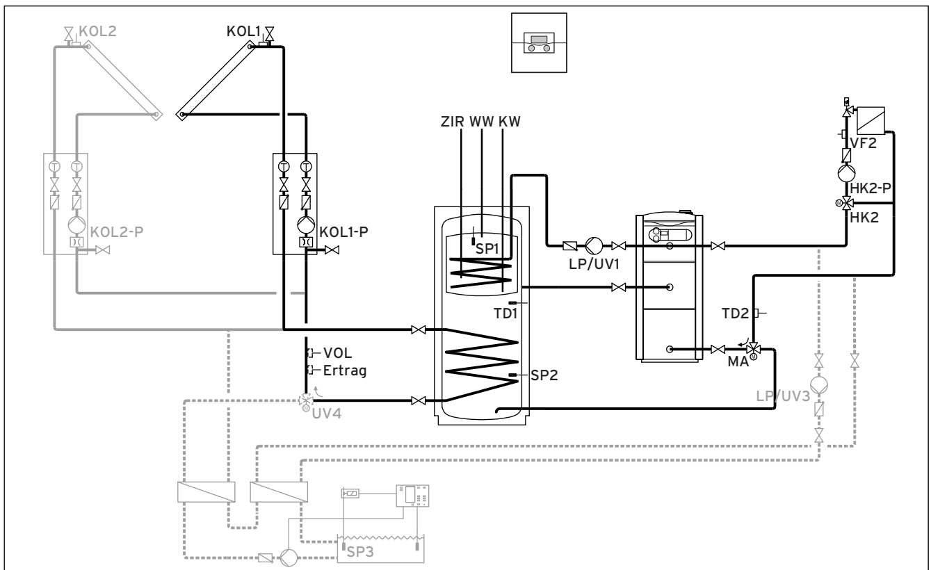
Fig. 5.9 Schéma hydraulique 3
