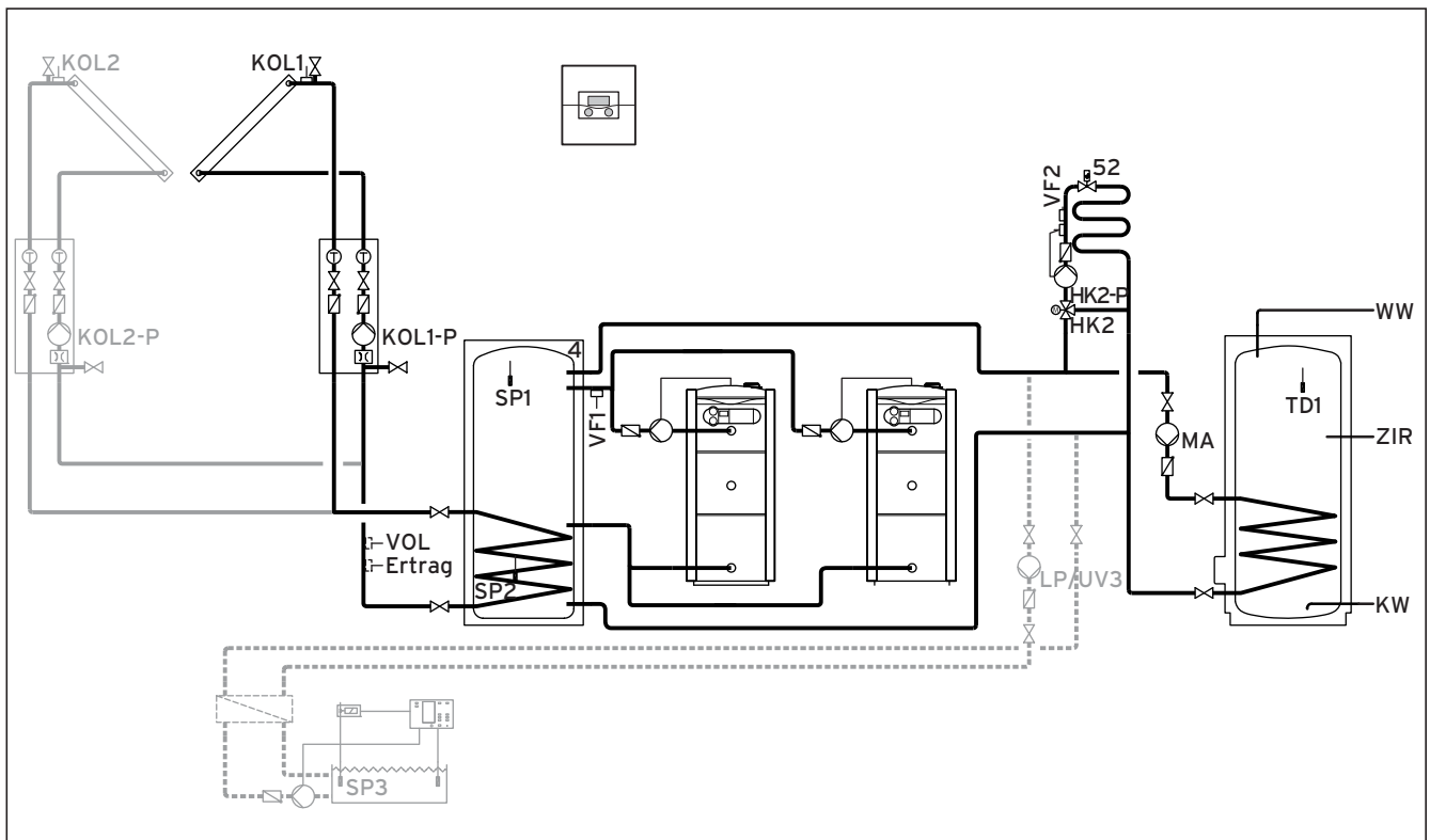
Fig. 5.31 Schéma hydraulique 7.2
