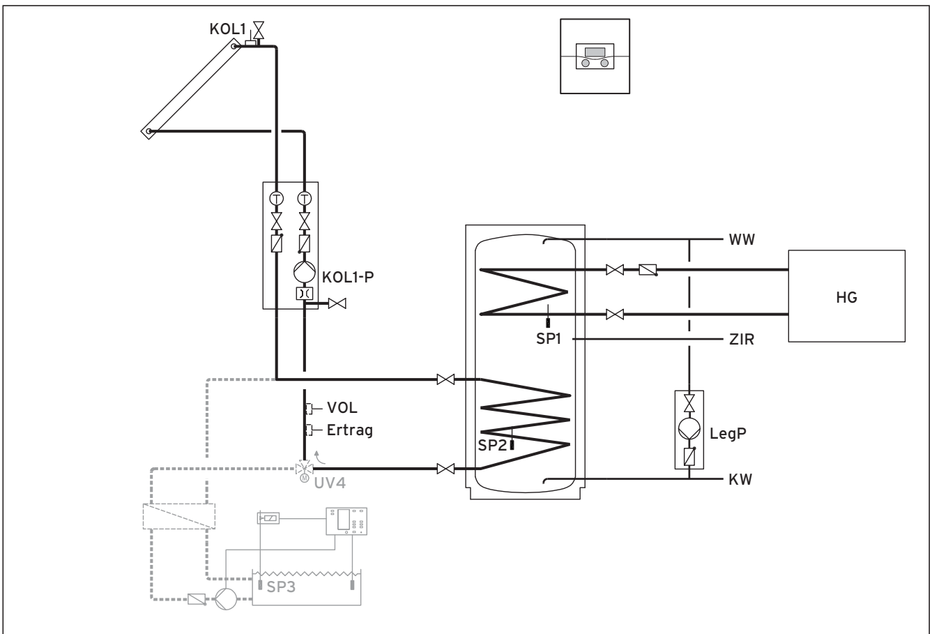
Fig. 5.11 Schéma hydraulique 3.1
