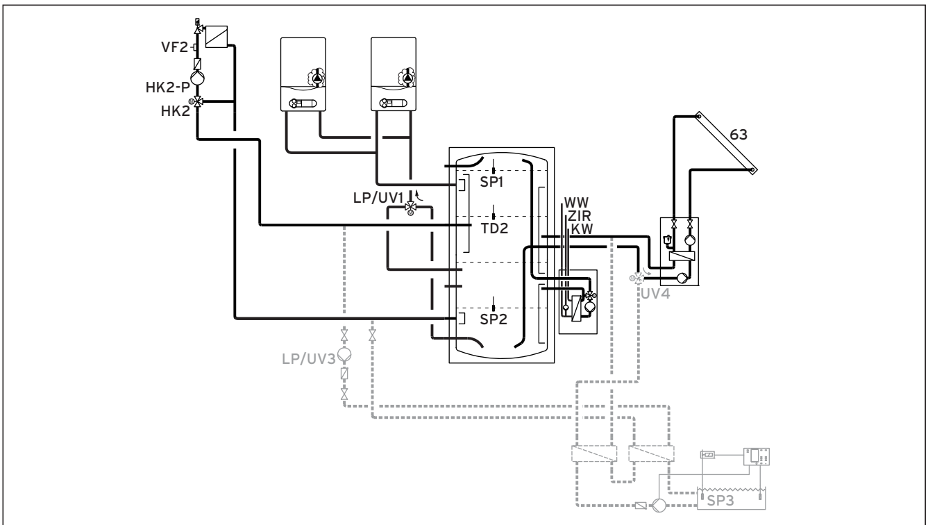
Fig. 5.39 Schéma hydraulique 9.3
