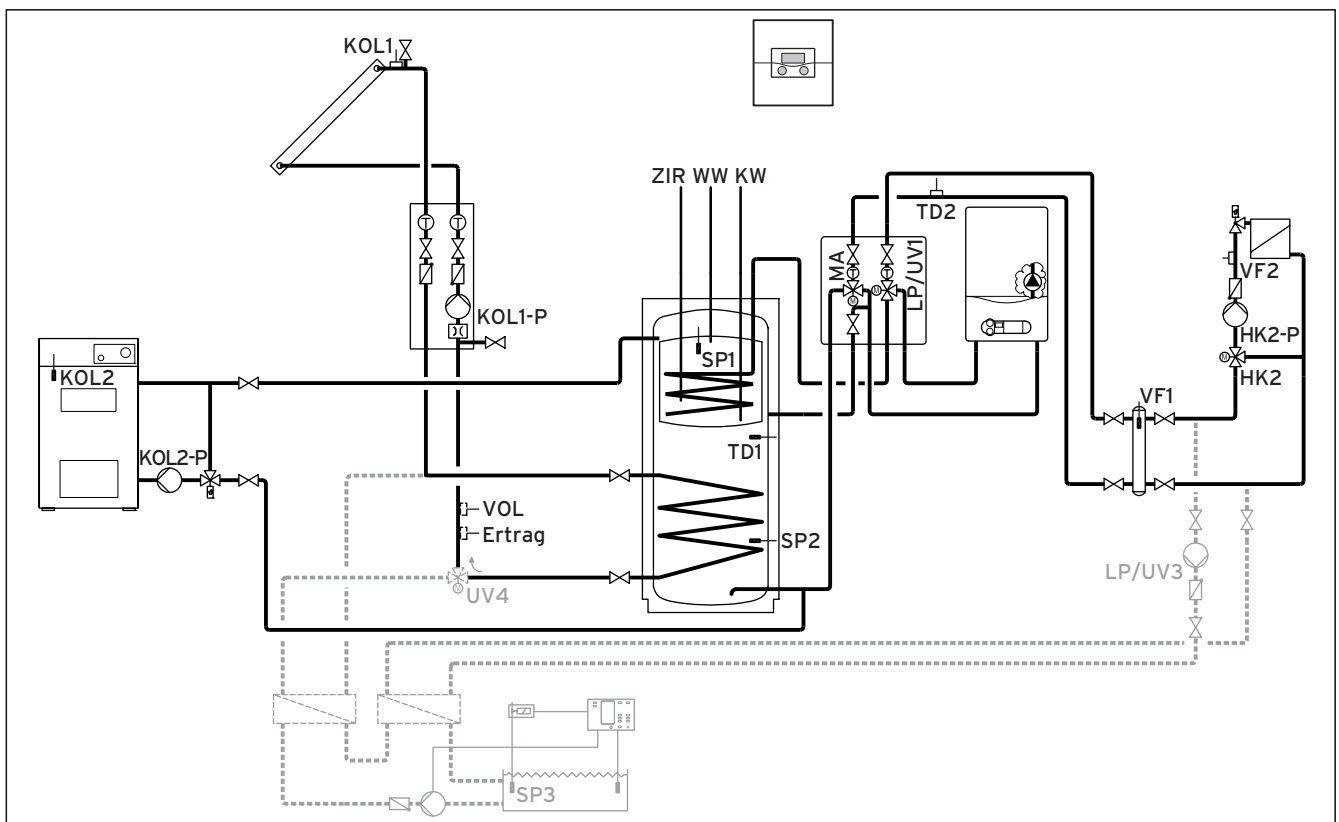
Fig. 5.5 Schéma hydraulique 2.1
