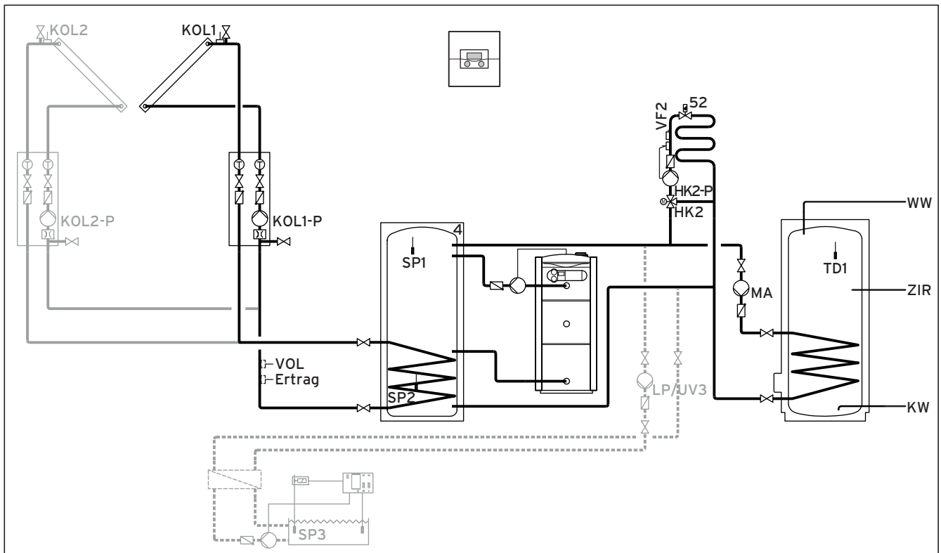
Fig. 5.29 Schéma hydraulique 7.1
