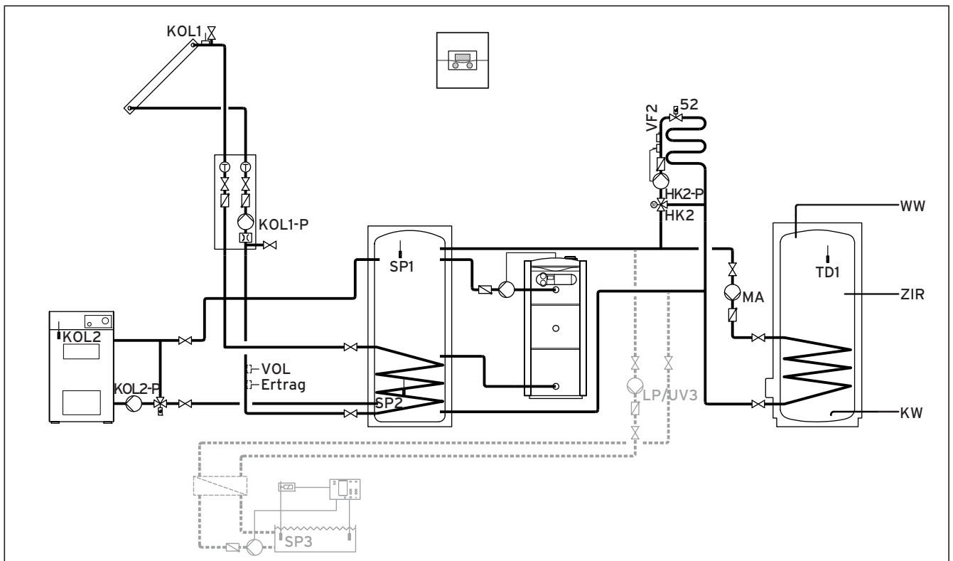
Fig. 5.33 Schéma hydraulique 8
