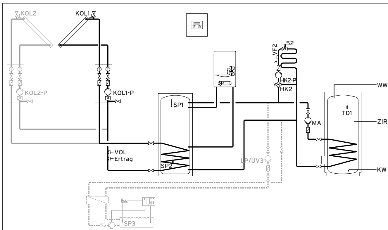
Fig. 5.23 Schéma hydraulique 5.1
