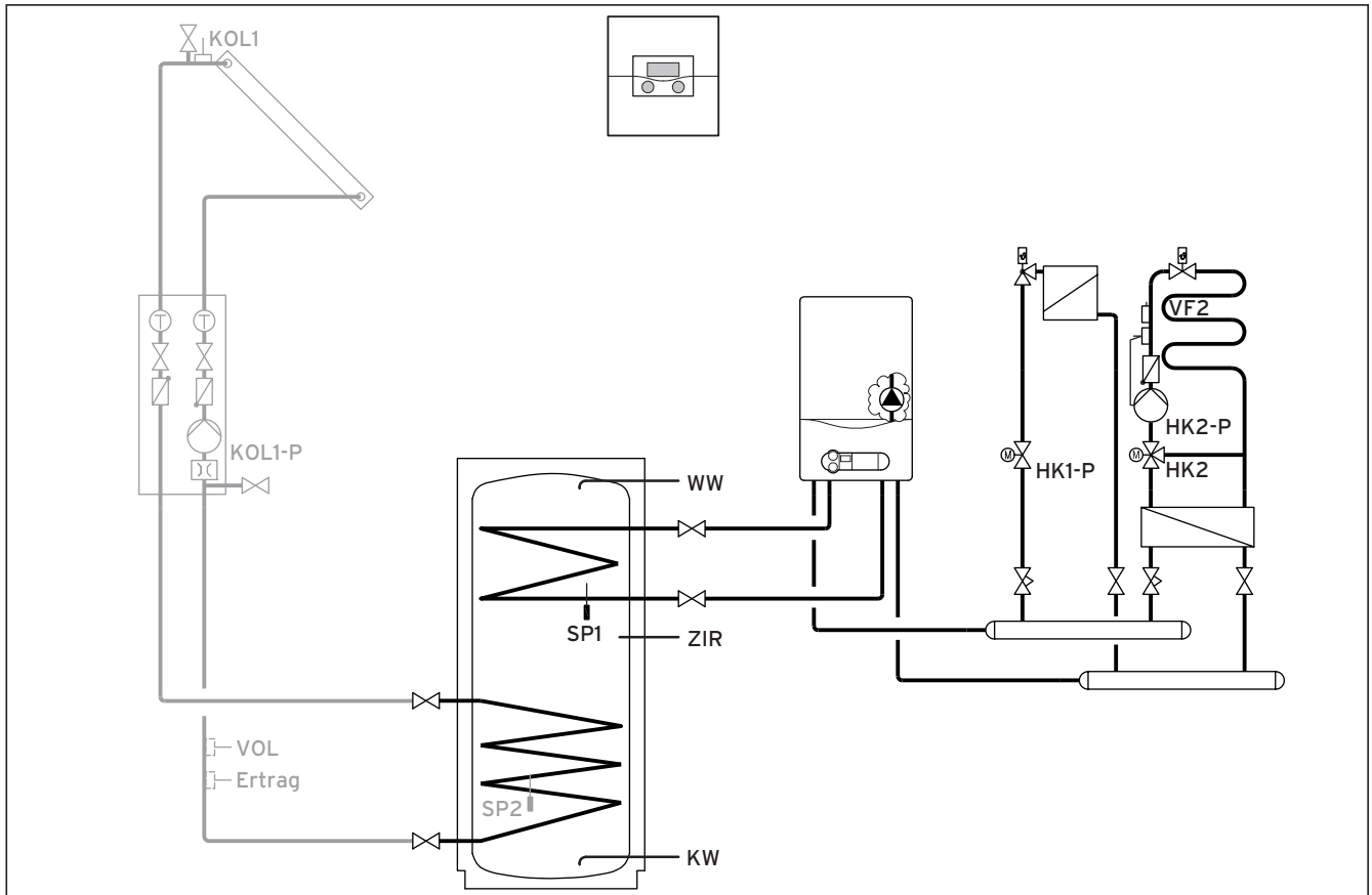
Fig. 5.15 Schéma hydraulique 3.3
