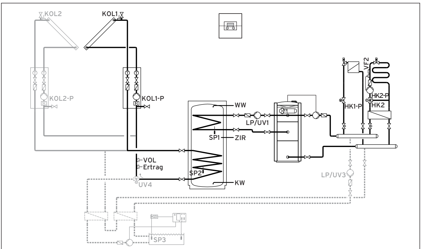
Fig. 5.17 Schéma hydraulique 3.4
